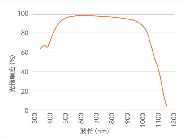
光谱响应
