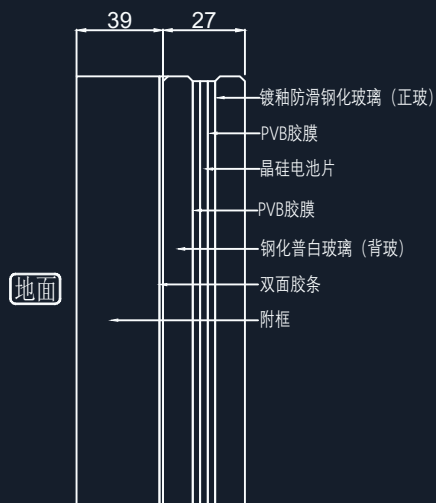
组件结构图
